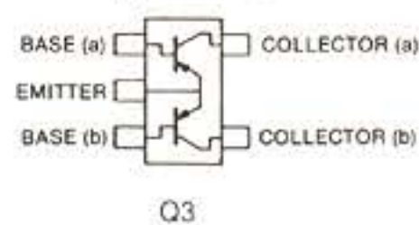
FMS1 (Symbol: SI)
