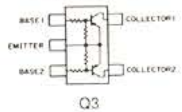
FMA2 (Symbol: A2)
