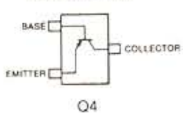
2SA1162 GR (Symbol: SG)
